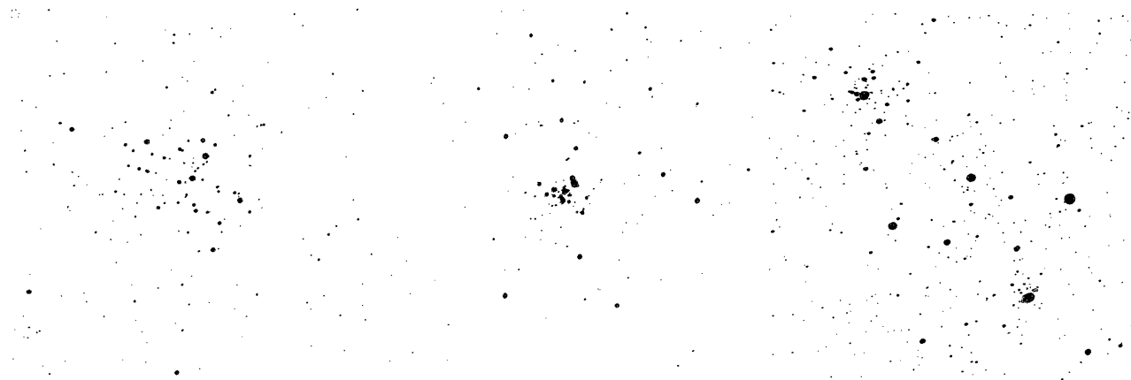
FIG. 10. 6405, MESSIER 6.
