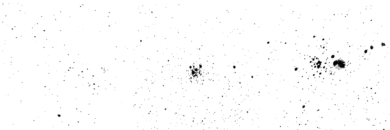
FIG. 13. 6633.
