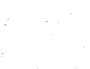
FIG. 9. 6712, CLUSTER.
