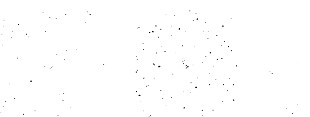
FIG. 29. 1952, CRAB NEBULA.
