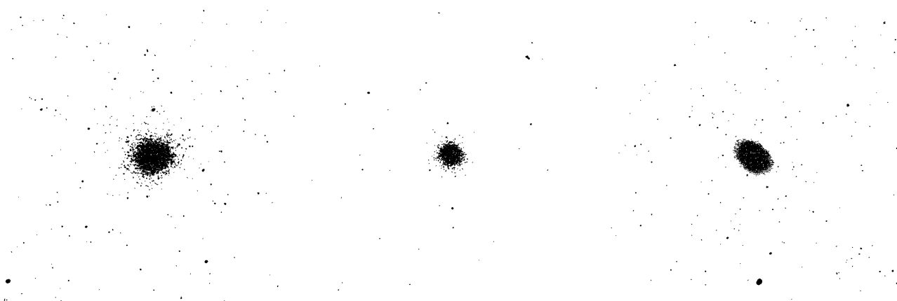
FIG. 16. 5139, \omega CENTAURI.
