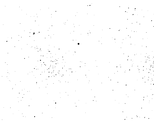
FIG. 26. 6494, MESSIER 23.
