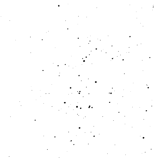
FIG. 2. 2632, PRAESEPE.
