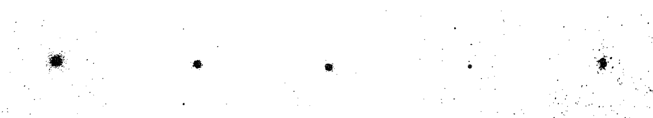
FIG. 19. 6205, HERCULES.
