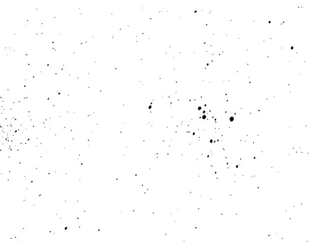
FIG. 27. 2437, MESSIER 46.
