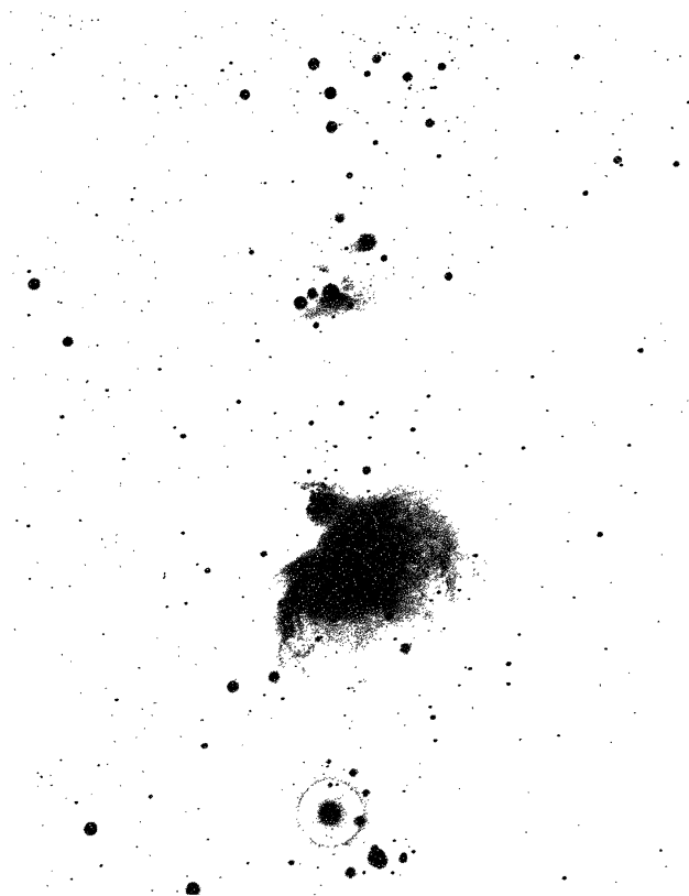
FIG. 24. 1976, ORION NEBULA. 1977. 1980. 1981.
