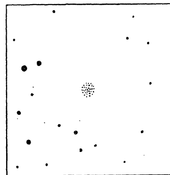
16^{\text{h}} 57^{\text{m}}.8 \quad -24^{\circ} 37'
