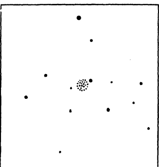
17^{\text{h}} 09^{\text{m}}.7 \quad -28^{\circ} 01'
