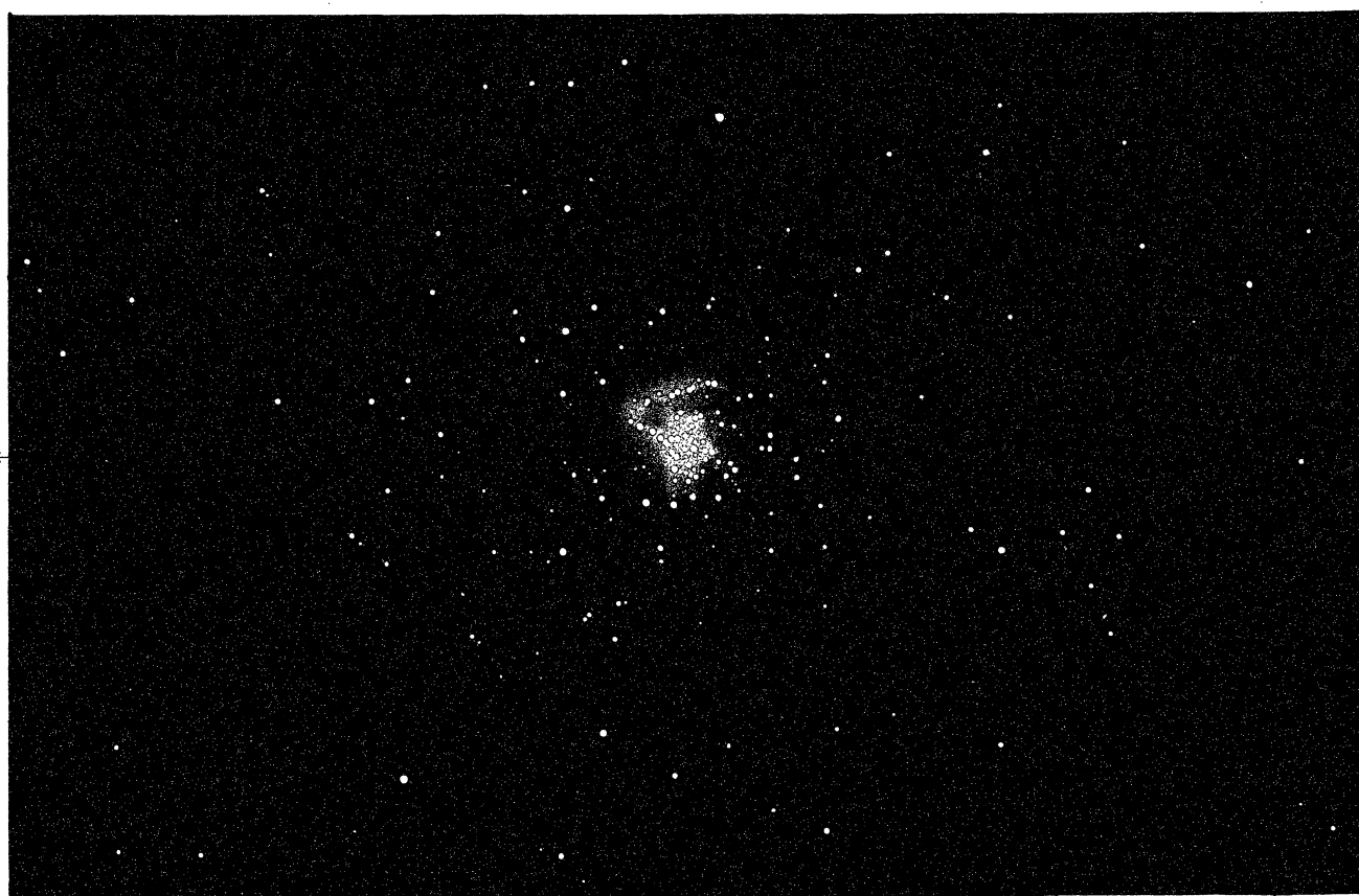
Nº Herschel Cat. 4294
