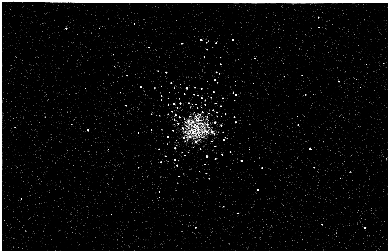
Nº Herschel Cat. 4230.
